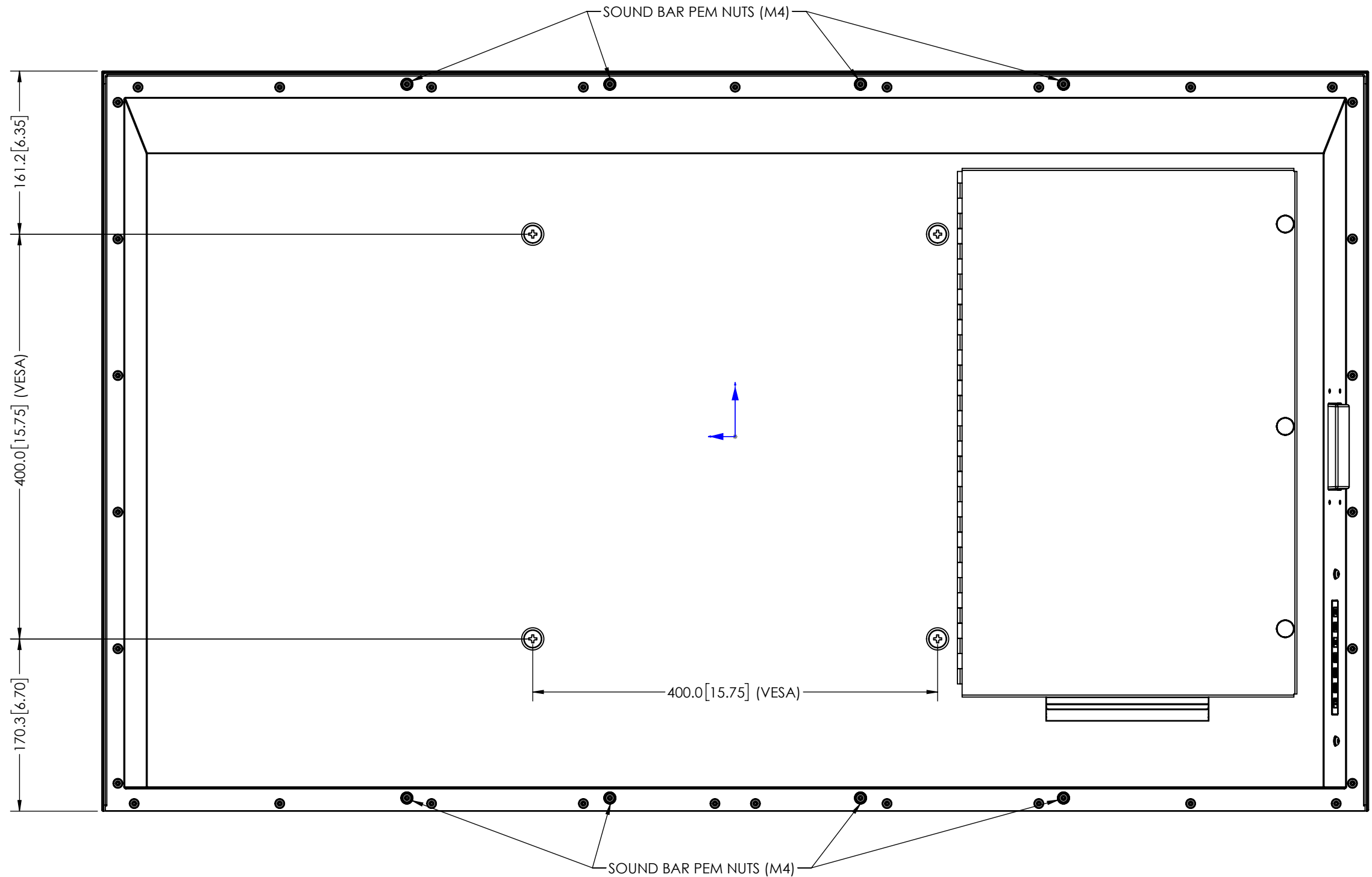
VIEW A-A
